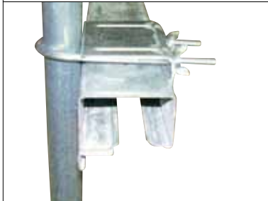
使用図
