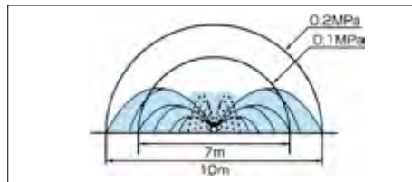
スミサンスイR露地ワイド散水イメージ図
