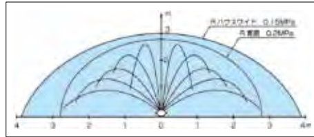
スミサンスイRハウスワイド散水イメージ図
