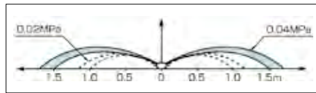
スミサンスイマルチ散水イメージ図
